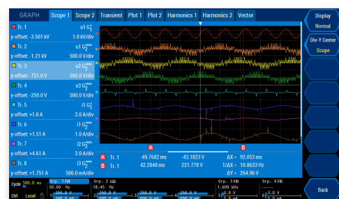
Darstellung der abgesteuerten Werte in zwei Scopes
